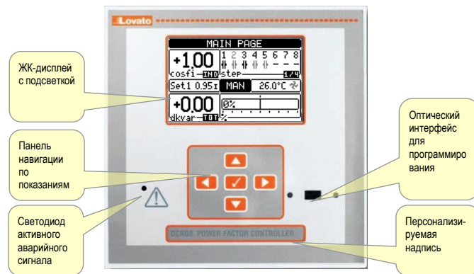
Передняя панель DCRG8
